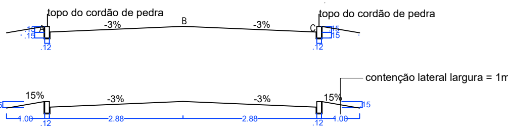
Contenção lateral com solo (apiloado)
