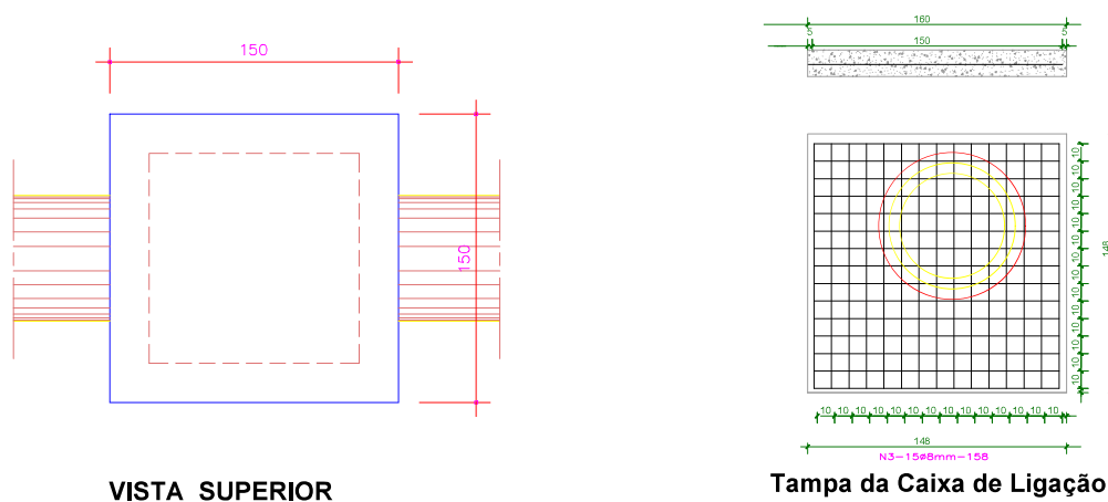
PLANTA BAIXA ESC.: 1:400 DETALHAMENTO DA CAIXA DE LIGAÇÃO
