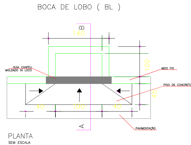
DETALHAMENTO DA BOCA DE LOBO
