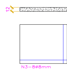
DETALHE TAMPA SUPERIOR E INFERIOR
