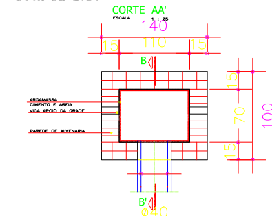
BOCA DE LOBO
